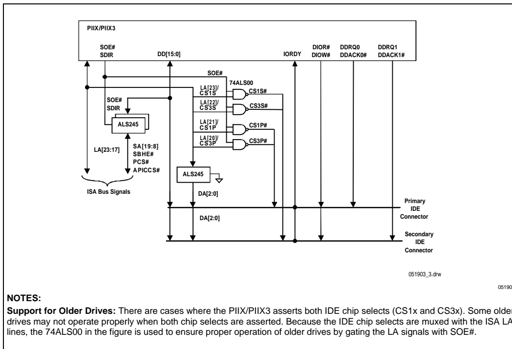
Figure 3. PIIX/PIIX3 IDE Interface
